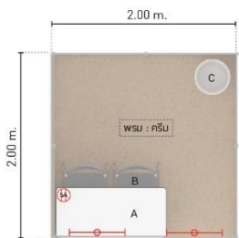
LAY-OUT-PLAN SCALE 1:50
